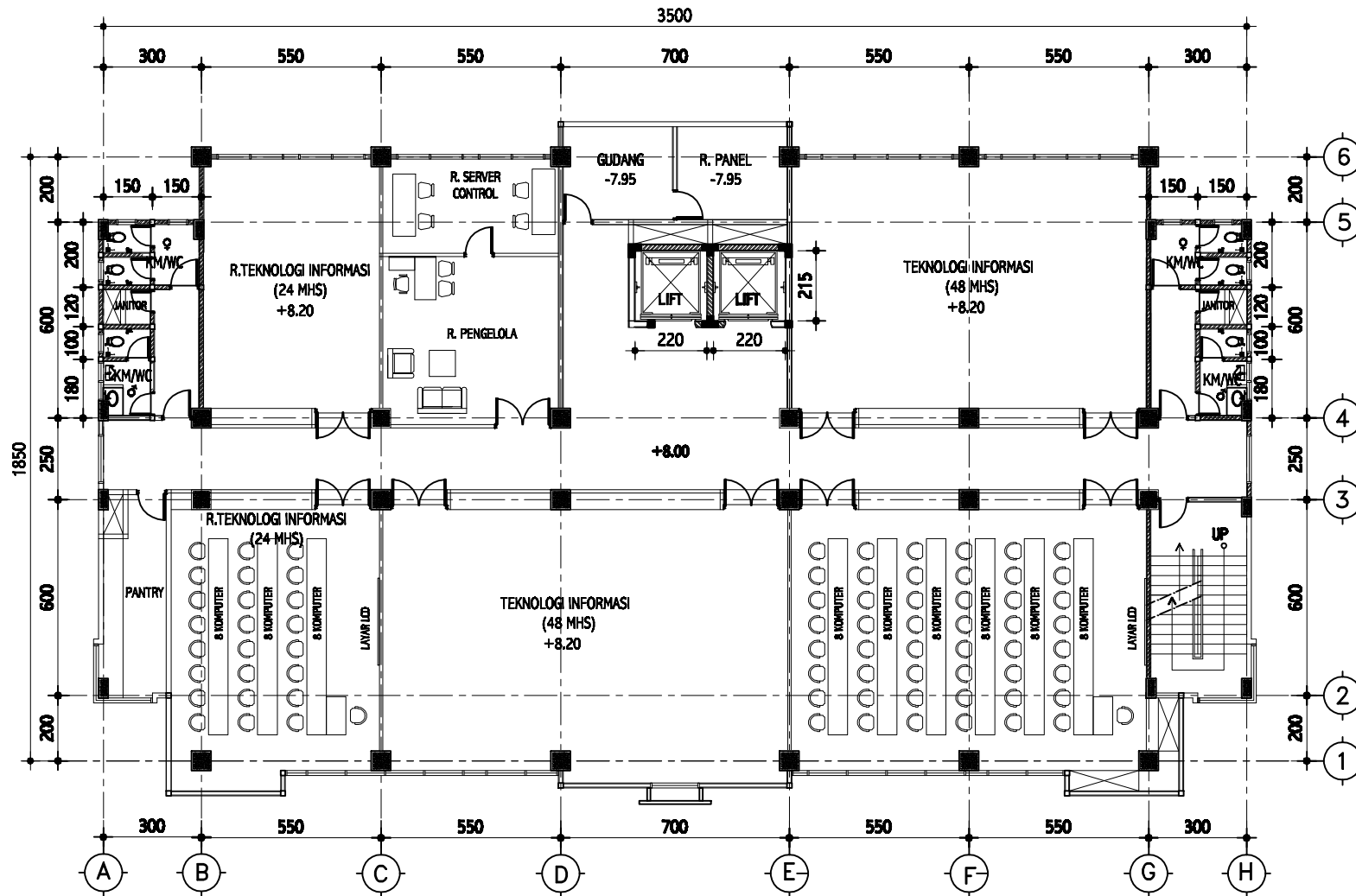
DENAH LT. 02 SKALA 1 : 150
