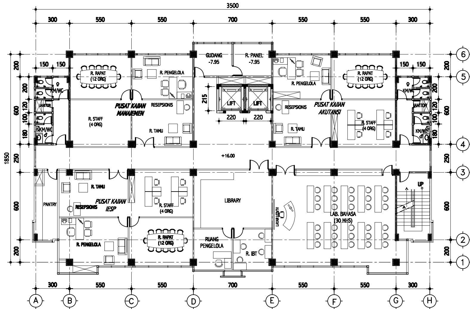
DENAH LT. 04 SKALA 1 : 150
