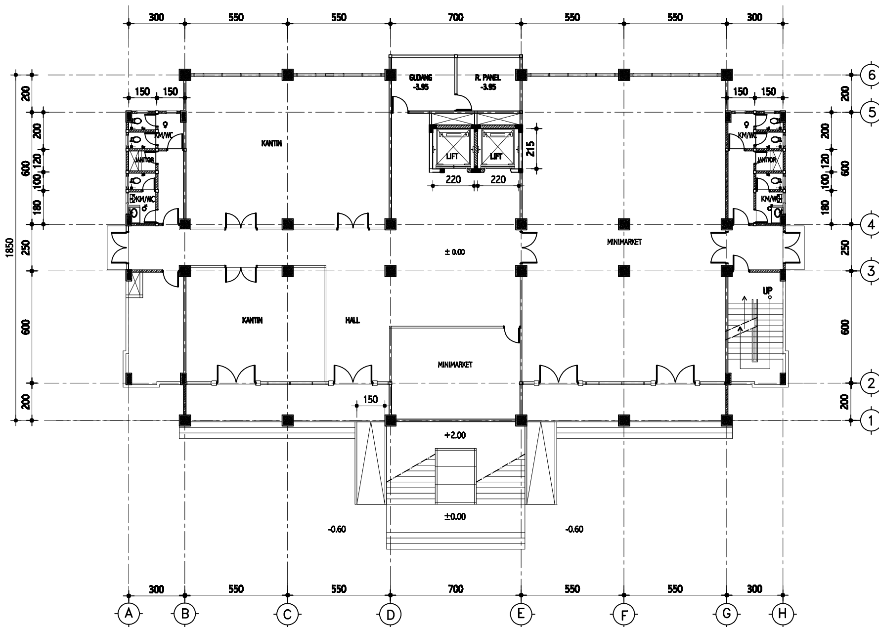
DENAH LT. DASAR
